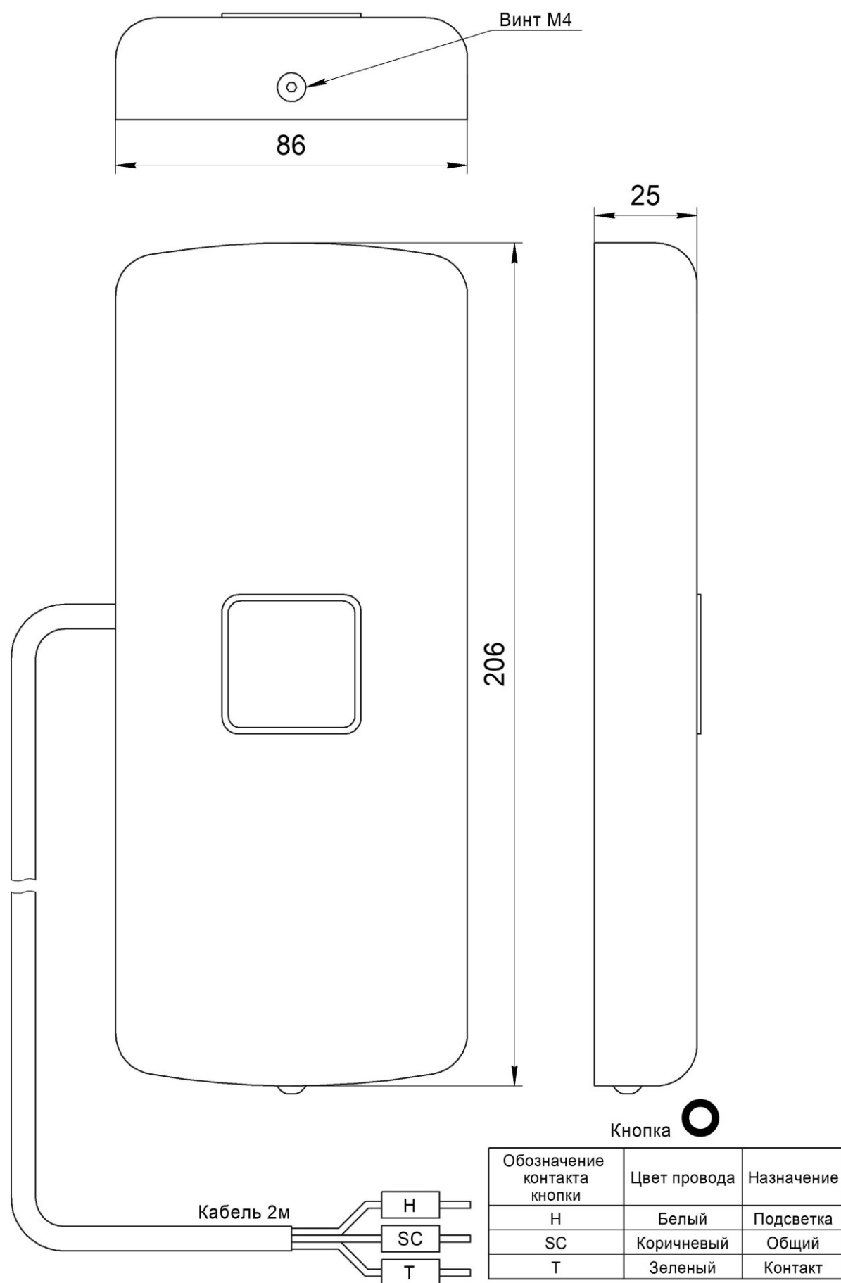
Рис.1 Внешний вид и габаритные размеры Вызывного поста ВП-1000-01
